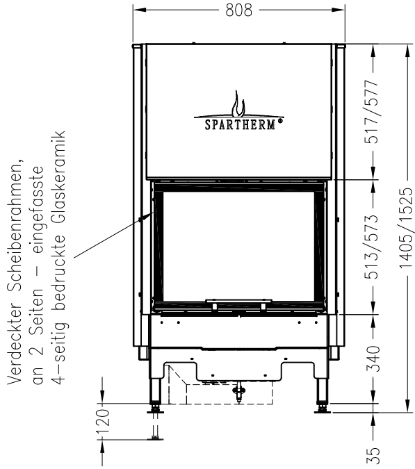
Vorderansicht M~1:20
